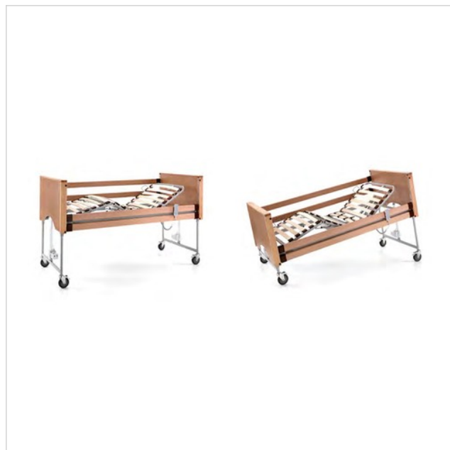
Regolazione altezza e posizione di Trendelenburg/contro-Trendelenburg
